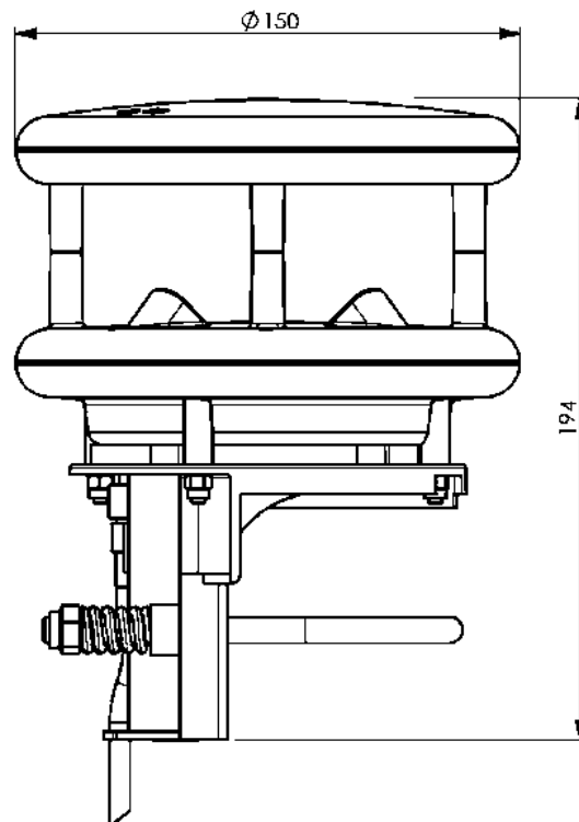
Рис. 21: WS200-UMB
