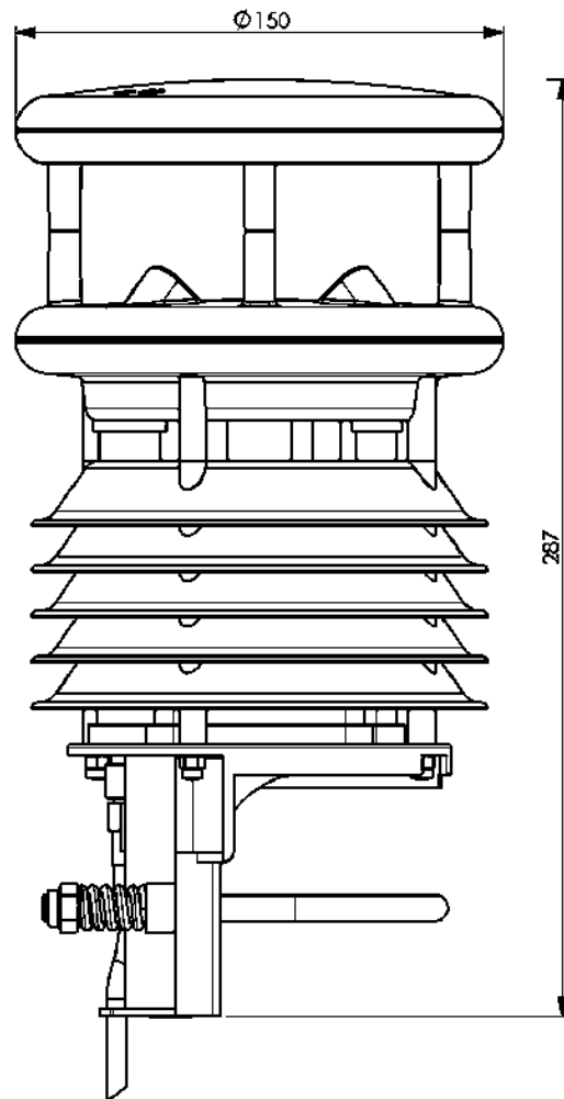
Рис. 26: WS500-UMB
